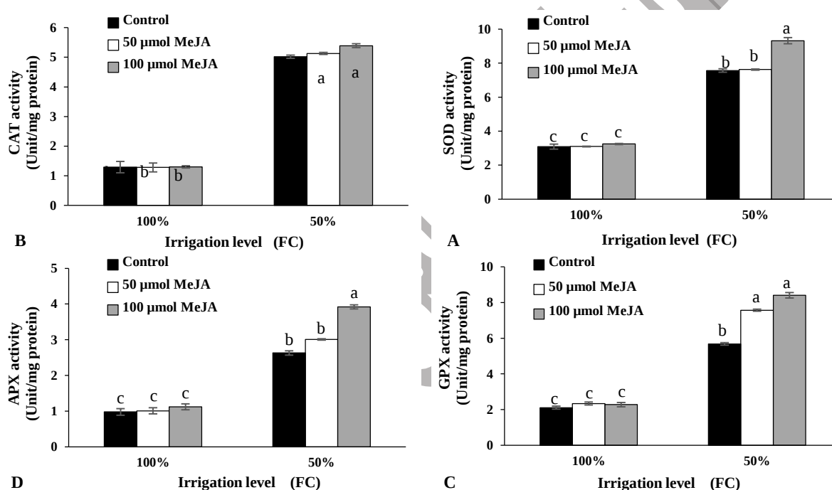
شکل ۱. تأثیر محلول پاشی متیل جاسمونات بر میزان فعالیت آنزیم‌های سوپراکسید دیسموتاز (A) (SOD)، کاتالاز (B) (CAT)، گاباکول پراکسیداز (C) (GPX) و آسکوربات پراکسیداز (D) (APX) در گیاه شاهی تحت شرایط آبیاری کامل و تنش کم‌آبی. (حروف مشابه نشان‌دهنده عدم وجود تفاوت معنی‌دار بر اساس آزمون LSD در سطح احتمال پنج درصد است)
