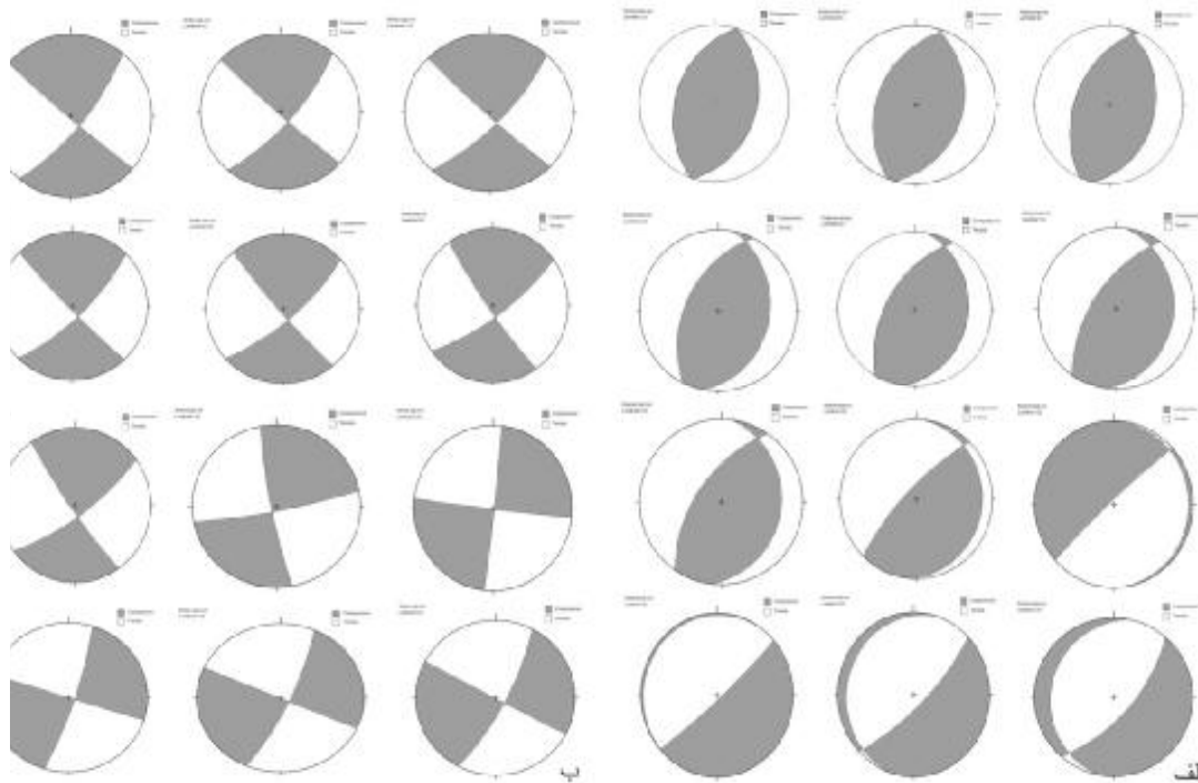
شکل 10. دو وجهی‌های عمود برهم مرتبط با الف گسلش نرمال و ب گسلش امتدادلغز در گستره مورد مطالعه.
