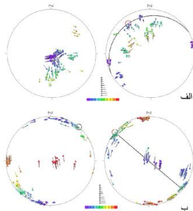
شکل 13- الف - نمایش موقعیت محورهای \sigma_3 و ب - نمایش موقعیت محورهای \sigma_1 استریوگرام حاصل از گسلش نرمال. ب - نمایش موقعیت محور \sigma_3 و شکل 13- الف - نمایش موقعیت محورهای \sigma_1 استریوگرام‌های سمت چپ موقعیت محور \sigma_1 استریوگرام حاصل از گسلش امتداد لغز \sigma_3 و \sigma_1 های طیف رنگین تغییرات شکل میدان از \sigma (نشانه دایره‌ای) را و استریوگرام‌های سمت راست موقعیت محور (رنگ بنفش) به کلوچه‌ای (رنگ سرخ) را نشان می‌دهد. دو کی
