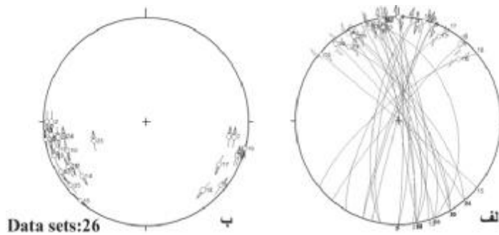
شکل 6. تصویر استریوگرافیک گسل‌های امتدادلغز در گستره مورد مطالعه. الف: تصویر استریوگرافیک خطوط لغزش مرتبط با این گسل‌ها ب: تصویر استریوگرافیک گسل‌های امتدادلغز که پیکان‌ها جهت حرکت فرادیواره را نسبت به فرودیواره نشان می‌دهد.
