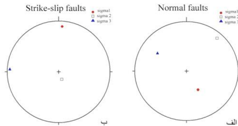
شکل 11. تصویر استریوگرافیک محورهای اصلی تنش براساس روش وارون سازی برای الف: گسلش نرمال ب: گسلش امتدادلغز.
