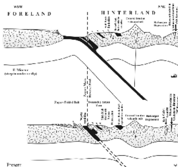
شکل 16. سیر تکاملی منطقه مورد مطالعه در لبه شمالی فروافتادگی رفسنجان به عنوان یک حوضه پشت کمبانی از کمربند ماگمایی ارومیه - دختر (Shahabpour, 2003)
