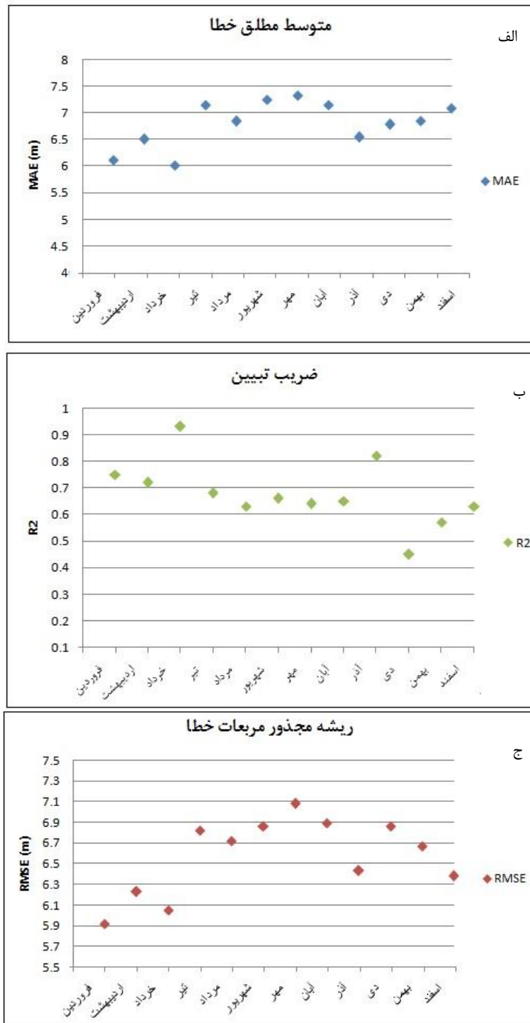
شکل ۲. تغییرات شاخص‌های ارزیابی مدل رگرسیون فازی امکانی در ماه‌های مختلف سال Fig 2. Goodness of fit statistics of fuzzy regression model in different months
