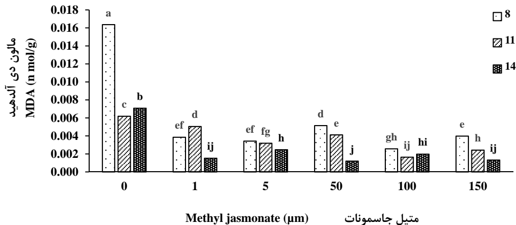
شکل ۷. اثر متیل جاسمونات بر مالون دی‌آلدئید کدو پوست کاغذی تحت تنش سرما. میانگین‌های دارای حروف مشابه بر اساس آزمون LSD فاقد اختلاف آماری معنی‌دار هستند.
