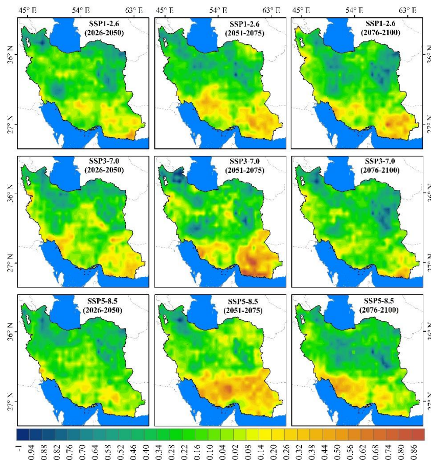
شکل ۳. پراکنش مکانی بی‌هنجاری‌های شدت خشکسالی در ایران برای افق‌های آینده نزدیک (۲۰۲۶-۲۰۵۰)، آینده میانی (۲۰۵۱-۲۰۷۵) و آینده دور (۲۰۷۶-۲۱۰۰). نسبت به دوره تاریخی (۱۹۹۰-۲۰۱۴). مبتنی بر برونداد CMIP6-MME تحت سناریوهای اجتماعی-اقتصادی SSP1-2.6 (خوش بینانه)، SSP3-7.0 (بدبینانه) و SSP5-8.5 (خیلی بدبینانه).
