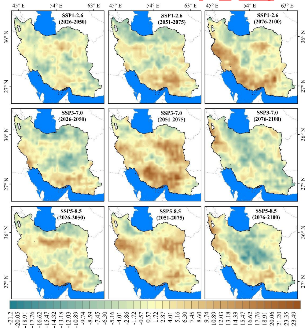
شکل ۴. پراکنش مکانی بی‌هنجاری‌های فراوانی خشکسالی در ایران برای افق‌های آینده نزدیک (۲۰۲۶-۲۰۵۰)، آینده میانی (۲۰۵۱-۲۰۷۵) و آینده دور (۲۰۷۶-۲۱۰۰). نسبت به دوره تاریخی (۲۰۱۴-۱۹۹۰). مبتنی بر برونداد CMIP6-MME تحت سناریوهای اجتماعی-اقتصادی SSP1-2.6 (خوش بینانه)، SSP3-7.0 (بدبینانه) و SSP5-8.5 (خیلی بدبینانه).
