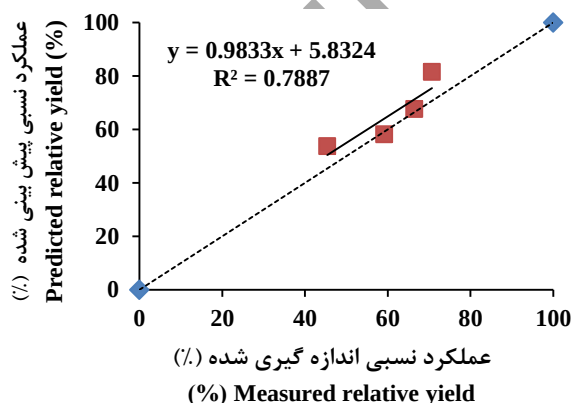
شکل ۶. نمودار صحت‌سنجی مدل باکتری سودوموناس Fig. 6. Validation diagram of the model Pseudomonas fluorescens treatment
