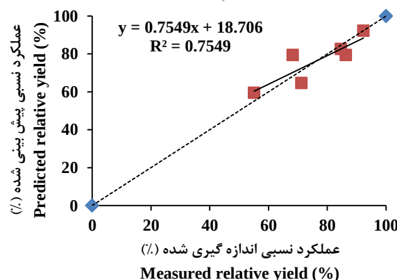
شکل ۳. نمودار واسنجی مدل تیمار قارچ تریکودرما Fig. 3. Model calibration diagram - Trichoderma harzianum treatment
