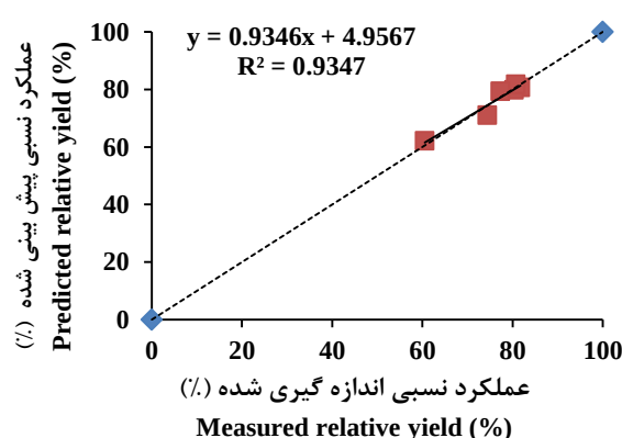
شکل ۴. نمودار صحت‌سنجی مدل - تیمار قارچ تریکودرما Fig. 4. Validation diagram of the model - Trichoderma harzianum treatment
