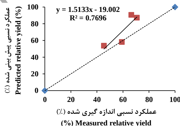
شکل ۵. نمودار واسنجی مدل - باکتری سودوموناس Fig. 5. Model calibration diagram - Pseudomonas fluorescens treatment
