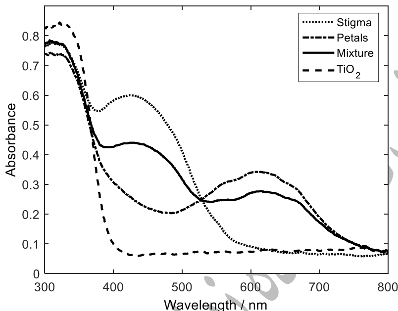
شکل ۳ طیف UV-Vis نفوذی-انعکاسی رنگ‌های مستخرج از پرچم، گلبرگ و مخلوط آن‌ها جذب شده بر روی نانوذرات آنتاز
