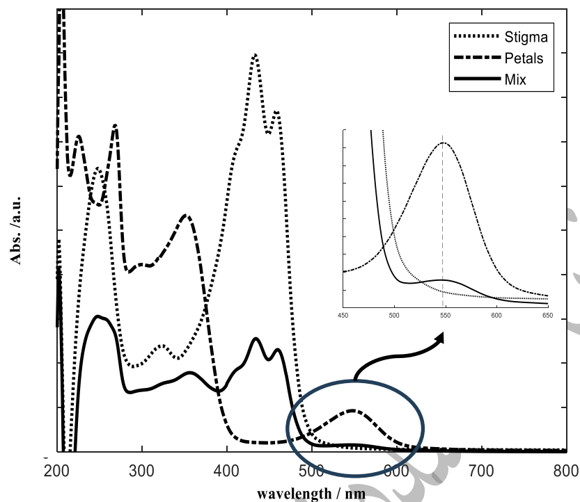
شکل ۱ طیف UV-Vis محلول رنگهای استخراج شده از پرچم و گلبرگ زعفران و مخلوط آنها
