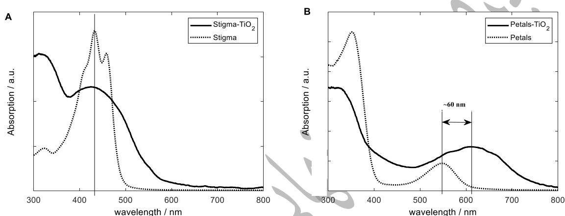
شکل ۴ مقایسه طیف UV-Vis رنگ‌های استخراج شده در محلول و رنگ‌های متصل‌شده به نانوذرات \text{TiO}_2 (A) رنگ استخراج شده از پرچم زعفران، و (B) رنگ استخراج شده از گلبرگ زعفران
