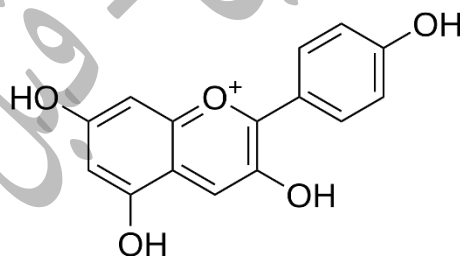
شکل ۲: مولکول پلارگونیدین
