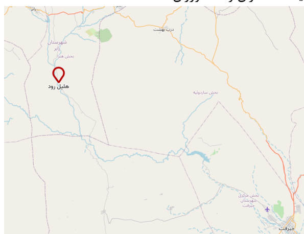
شکل ۱. تصویر هوایی منطقه هلیل‌رود
