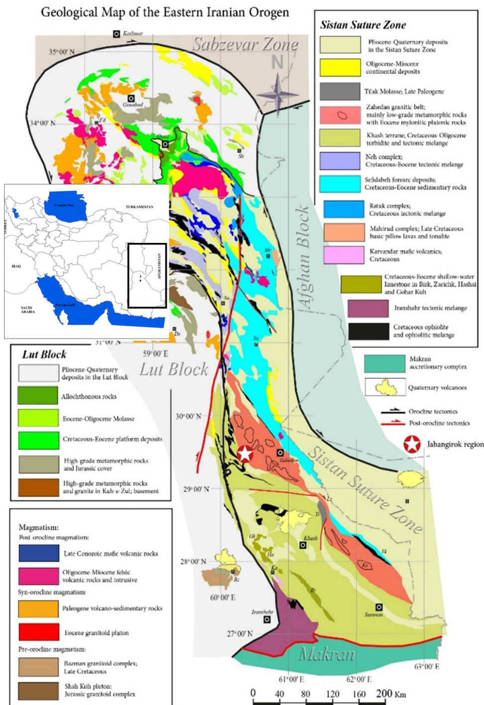
شکل ۱) مهمترین واحدهای تکتونیکی سازنده زمین‌شناسی شرق ایران (Bagheri and Damani Gol, 2020).
