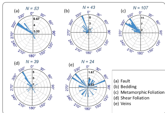
شکل ۱۱) نمودارهای گل سرخی عناصر ساختاری برداشت شده در منطقه جهانگیروک شمالی و جنوبی.
