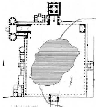
شکل ۳: پلان بخش‌های معماری کاخ آباکان، دوره ایلخانی، تخت سلیمان (Mousavi, 2021 :45)
