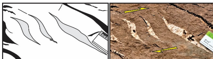
شکل ۵: شکستگی‌های کششی هلالی شکل که در پهنه برشی راستگرد تشکیل شده‌اند.
