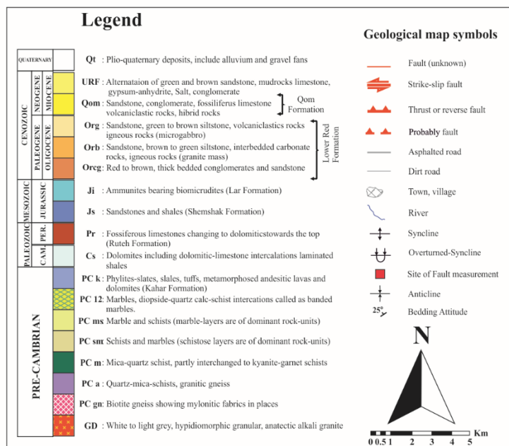
شکل ۲) نقشه زمین شناسی گستره ماهنشان که بر اساس برگه زمین شناسی ۱:۱۰۰۰۰۰ ماهنشان (لطفی، ۱۳۸۰)، سنجش از دور و مشاهدات صحرائی توسیم شده است.
