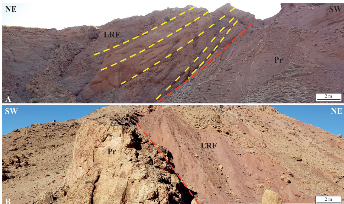
شکل ۴) A. چینه‌های رشدی در واحد Or cg واقع در تقادیس قزله‌بالا که روی آهک پرمین با شیب کمتر نهشته شده است. B. ناپوستگی سازند قم بر روی مجموعه دگرگونی تکاب و سازند قم روی سازند سرخ زیرین (واحد Or cg ) قرار گرفته است. خط چین زرد لایه‌بندی و خط چین قرمز ناپوستگی را نشان می‌دهد.
