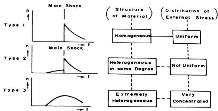
شکل ۶: الگوهای مختلف پراکندگی پیش لرزه‌ها و پس لرزه‌ها همراه با زمان و رابطه آنها با نوع ساختار مواد تشکیل دهنده محیط و نحوه پراکندگی تنش‌های خارجی اعمالی (Mogi, 1963).
