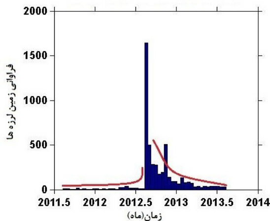
شکل ۷: الگوی زمان-فراوانی زمین لرزه‌های اهر-ورزقان
