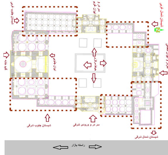
تصویر ۳: پلان بخش‌های مختلف مسجد امام (ره) بروجرد (آرشیو اداره میراث فرهنگی شهرستان بروجرد).
